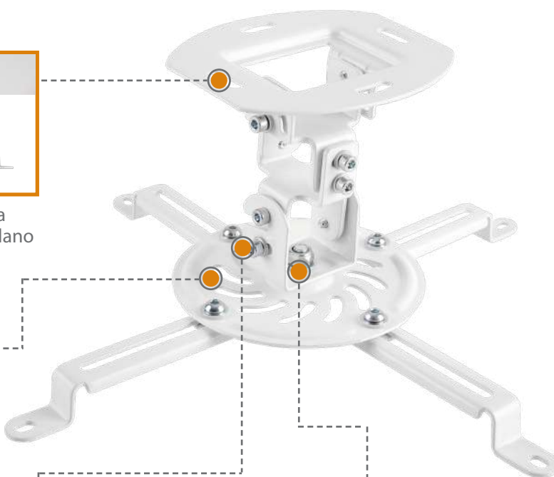
Araña ajustable a proyectores de diferentes tamaños.
